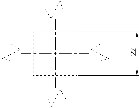
开孔尺寸(Cut Out)
