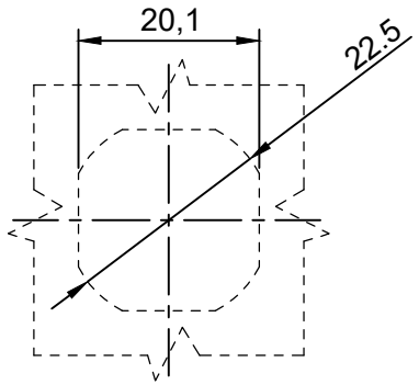
开孔尺寸(Cut Out)
