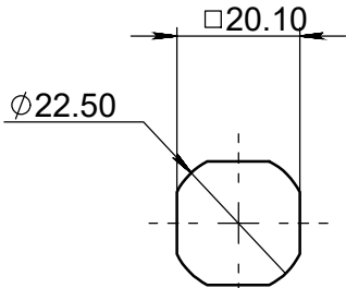
开孔尺寸(Cut Out)
