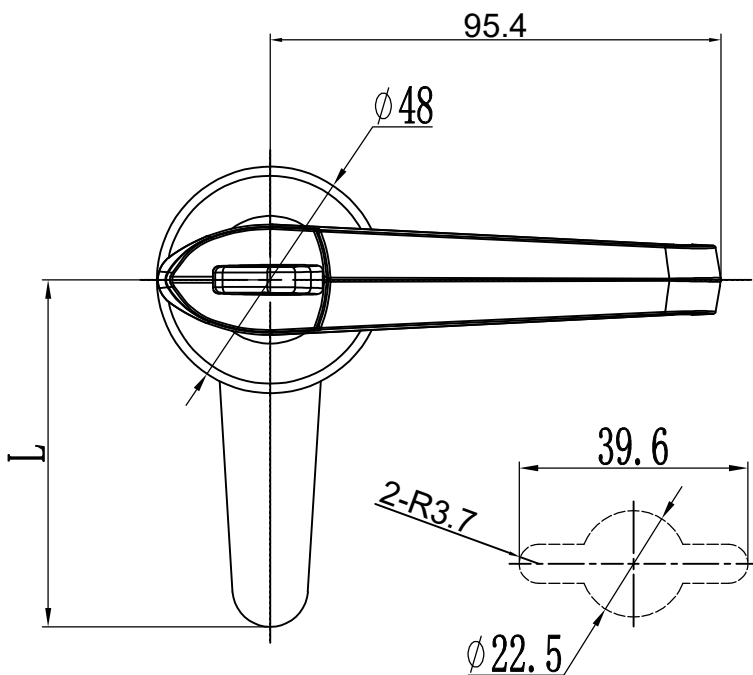
开孔尺寸
