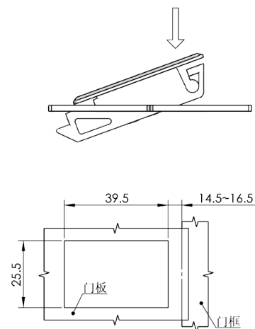
开孔尺寸 Cut out
