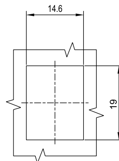
开孔尺寸 cut out
