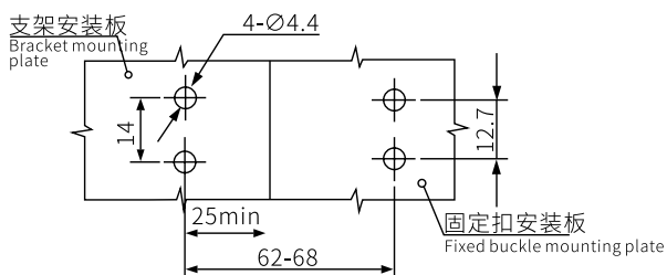
开孔尺寸 Cut out
