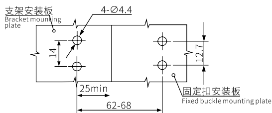
开孔尺寸 Cut out
