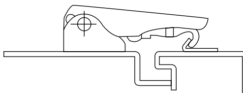
无防松扣型 Non-locking type
