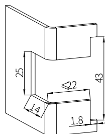
开孔尺寸 Panel cutout
